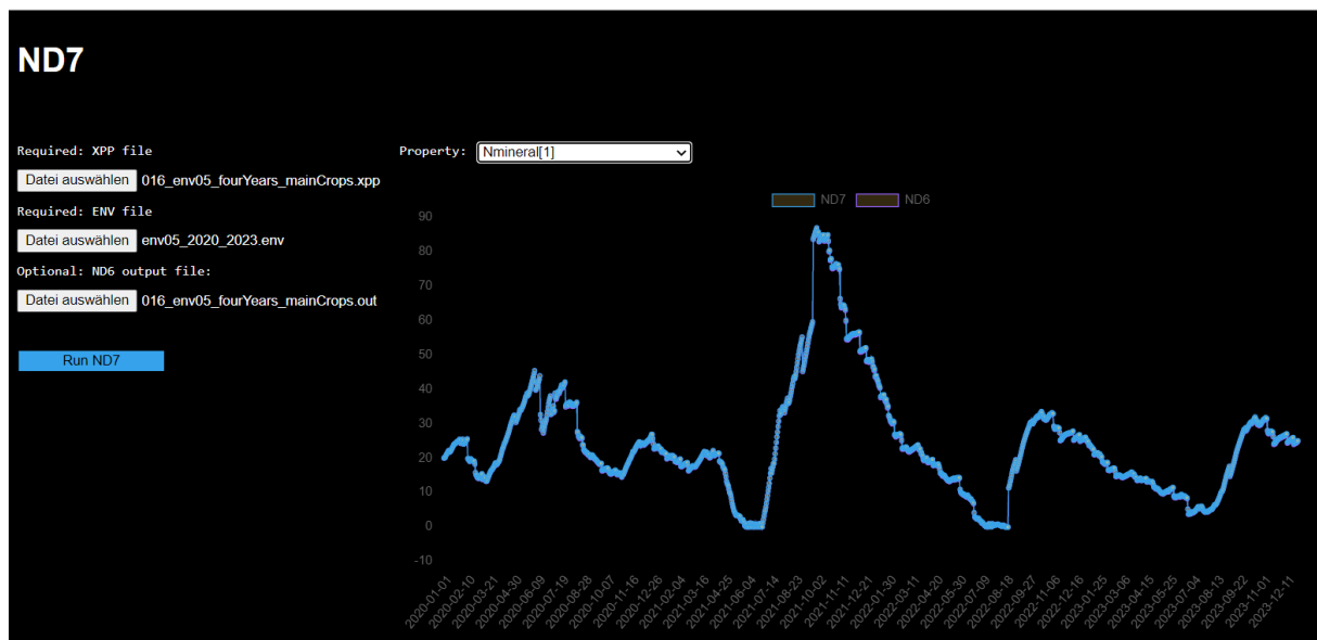
Abbildung 2.2-7: Nutzeroberfläche und Test Schnittstelle zur Überprüfung des neuen Rechenkerns. Die beiden Zeitlichen N_{\min} Verläufe für NDICEA 6 (pink) und NDICEA 7 (blau) liegen genau übereinander.
