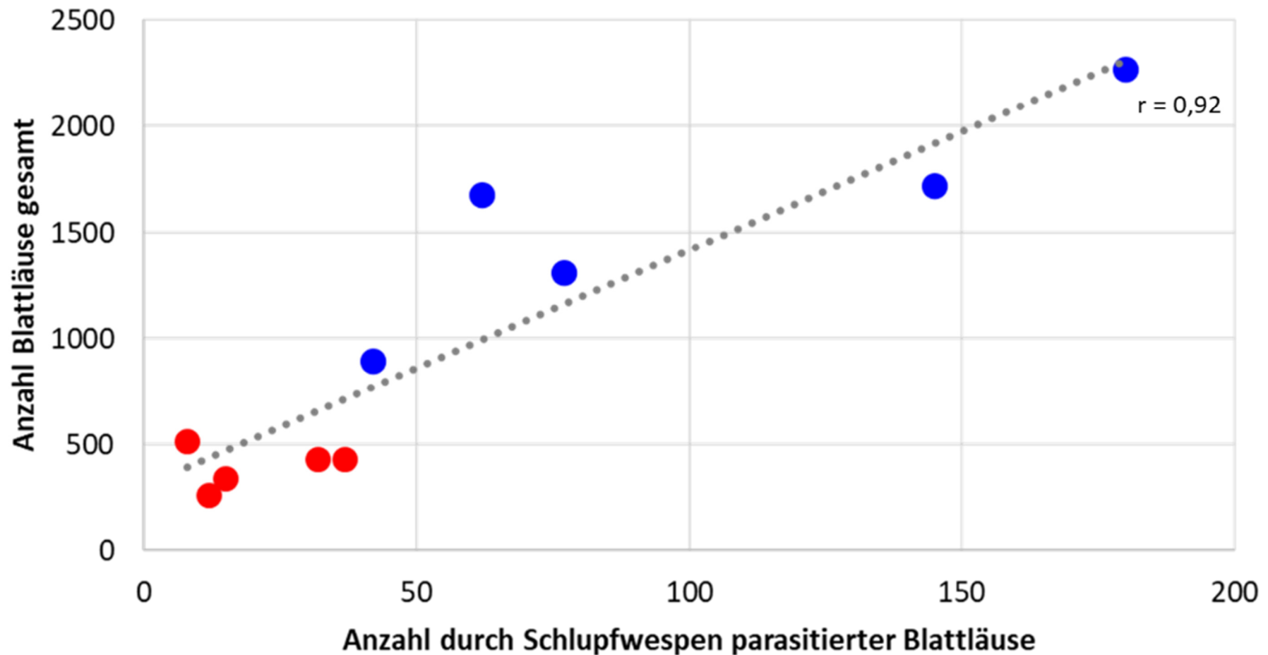
Beziehung zwischen Gesamtanzahl an Blattläusen und der Anzahl der durch Schlupfwespen parasitierter Blattläuse - Sortenversuch Niederkassel 2022 (n = 5 Sorten, ohne Insektizid: blau und mit Insektizid: rot)
